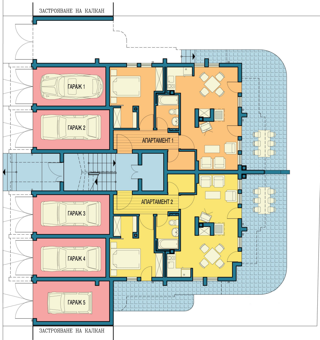
РАЗПРЕДЕЛЕНИЕ ПЪРВИ ЕТАЖ М 1:100
