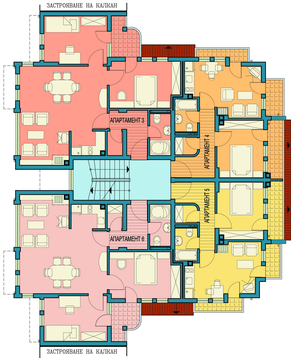
РАЗПРЕДЕЛЕНИЕ ВТОРИ ЕТАЖ М 1:100
