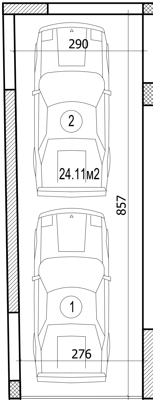
Гараж 27.33M2
