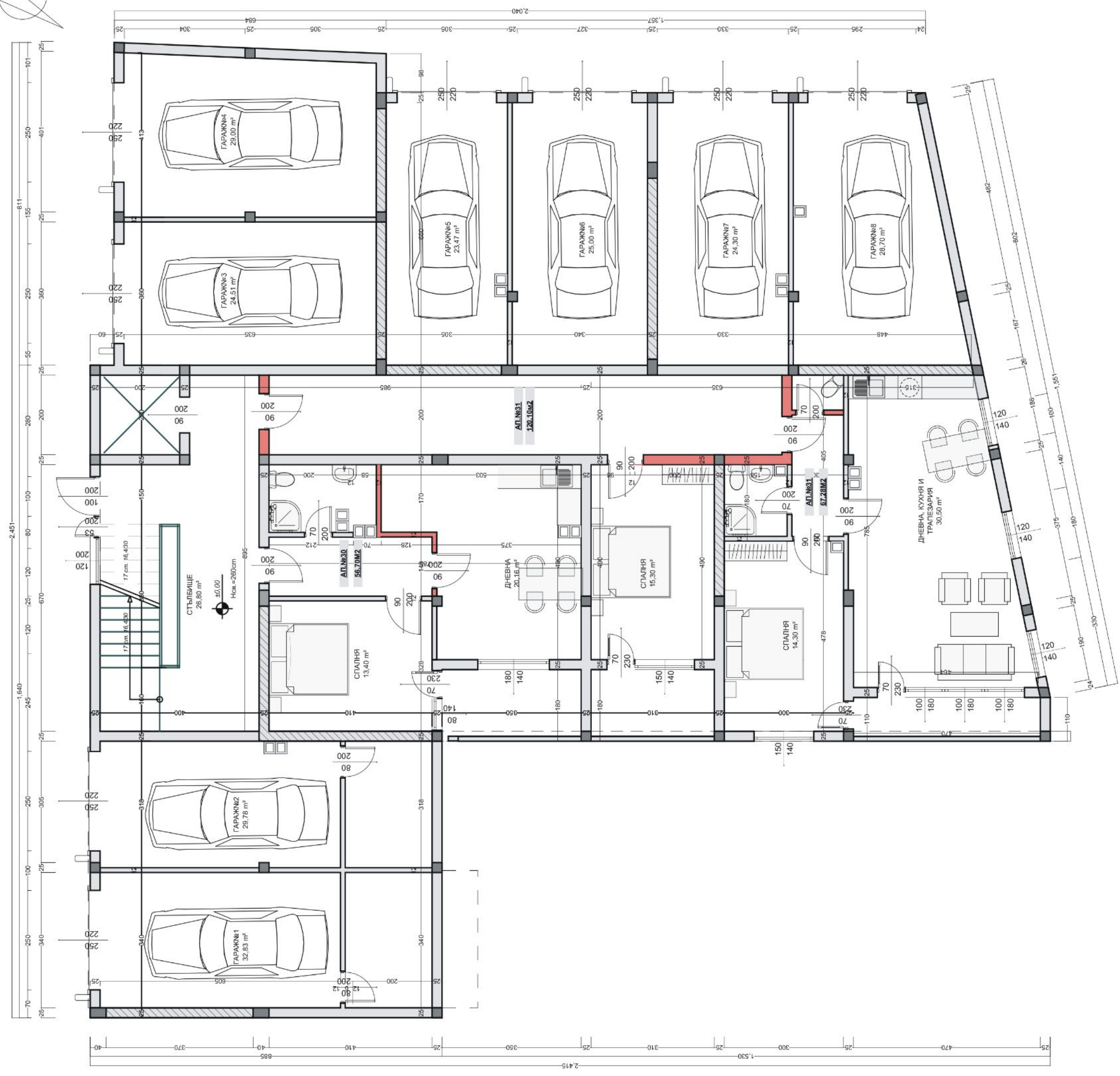
РАЗПРЕДЕЛЕНИЕ КОТА +0,00
