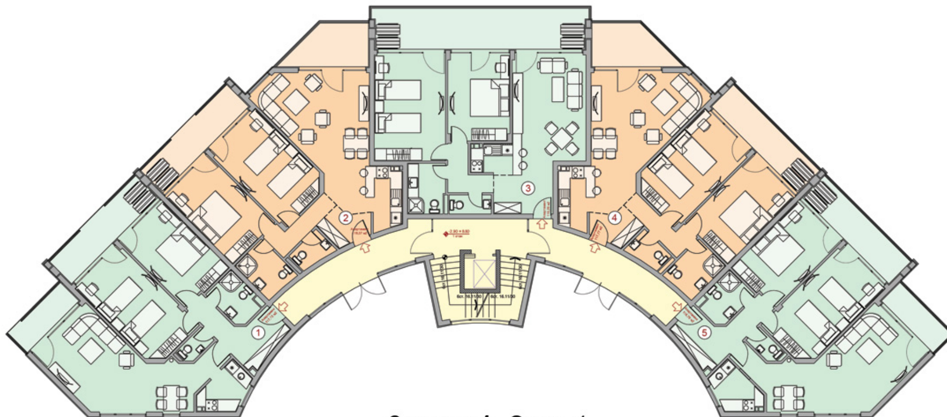
Здание 1 Этаж 1
