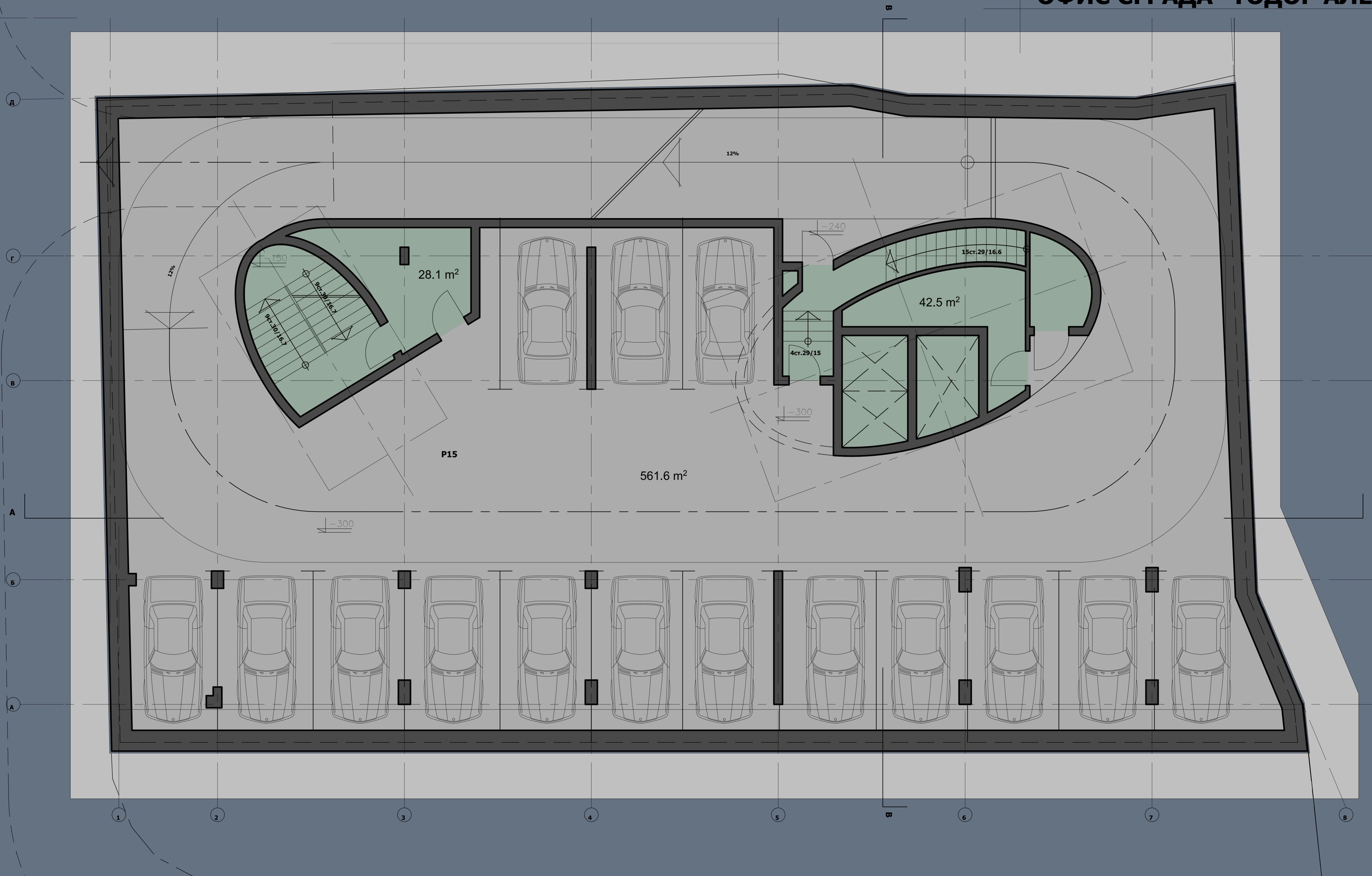
РАЗПРЕДЕЛЕНИЕ ПЪРВИ СУТЕРЕН М1:50 /кота -300/
