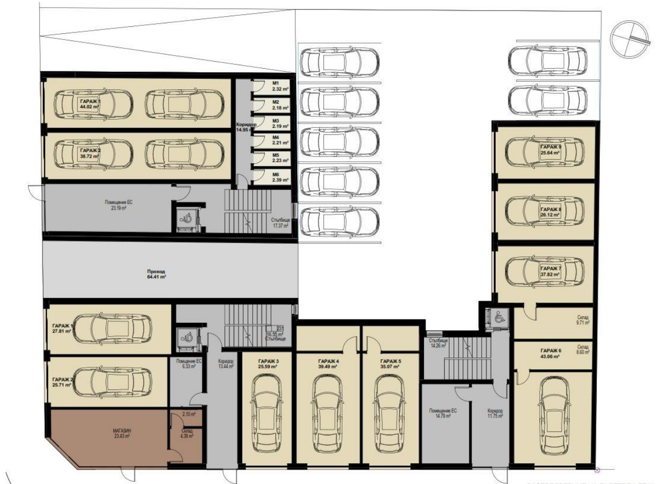
РАЗПРЕДЕЛЕНИЕ НА ПАРТЕРЕН ЕТАЖ
