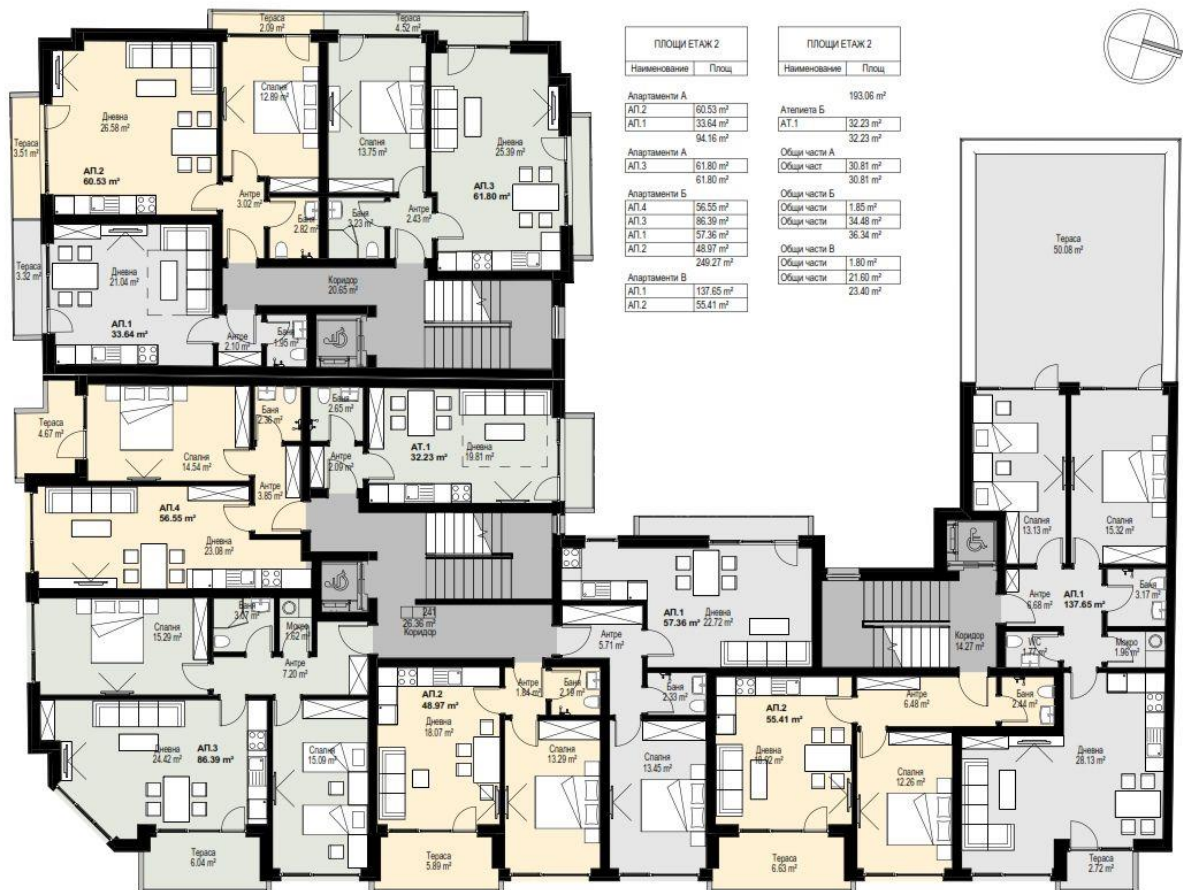
РАЗПРЕДЕЛЕНИЕ НА ВТОРИ ЕТАЖ
