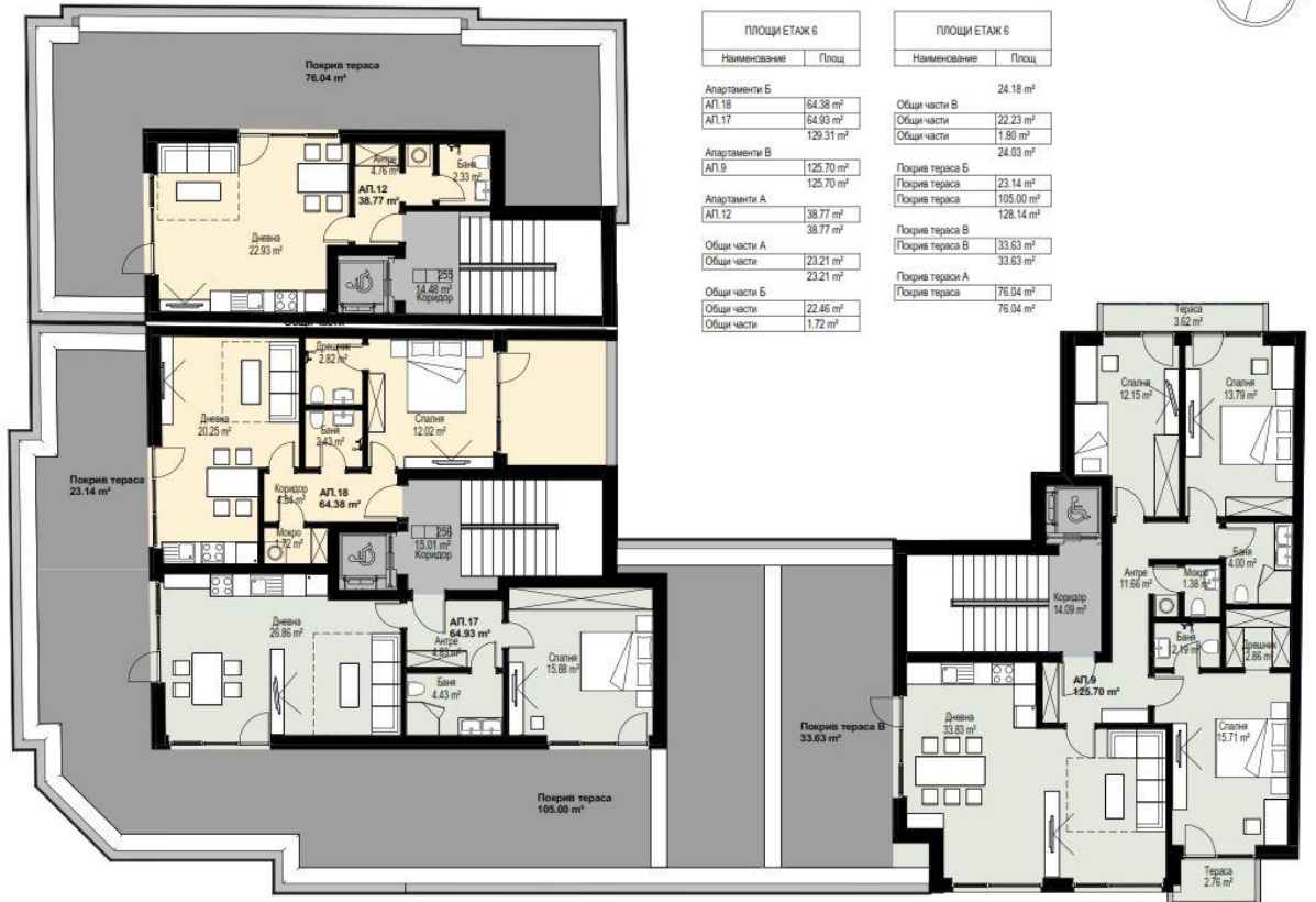
РАЗПРЕДЕЛЕНИЕ НА ШЕСТИ ЕТАЖ
