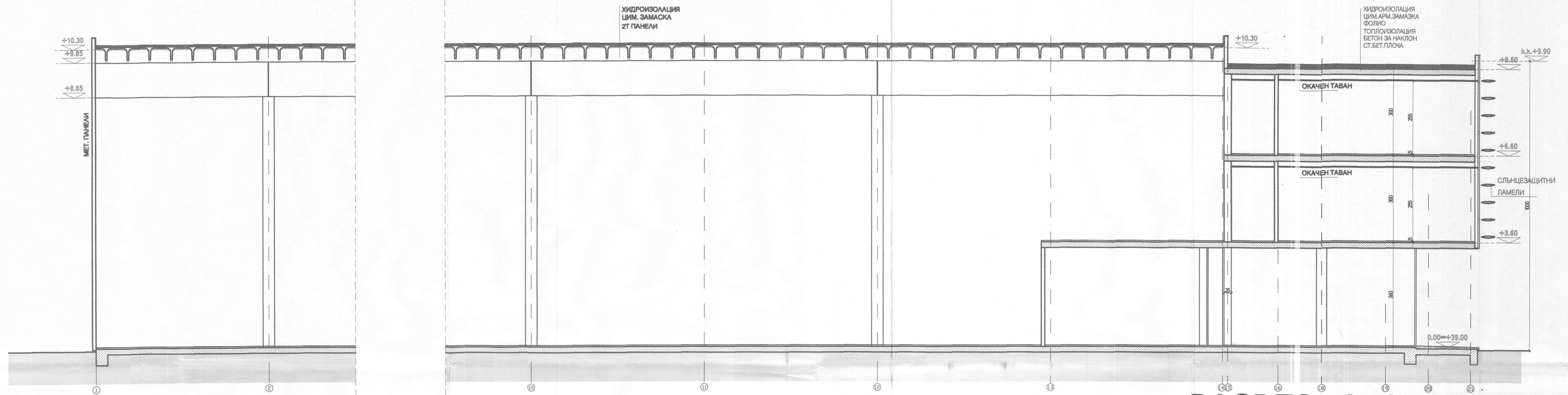
РАЗРЕЗ А-А М 1:75
