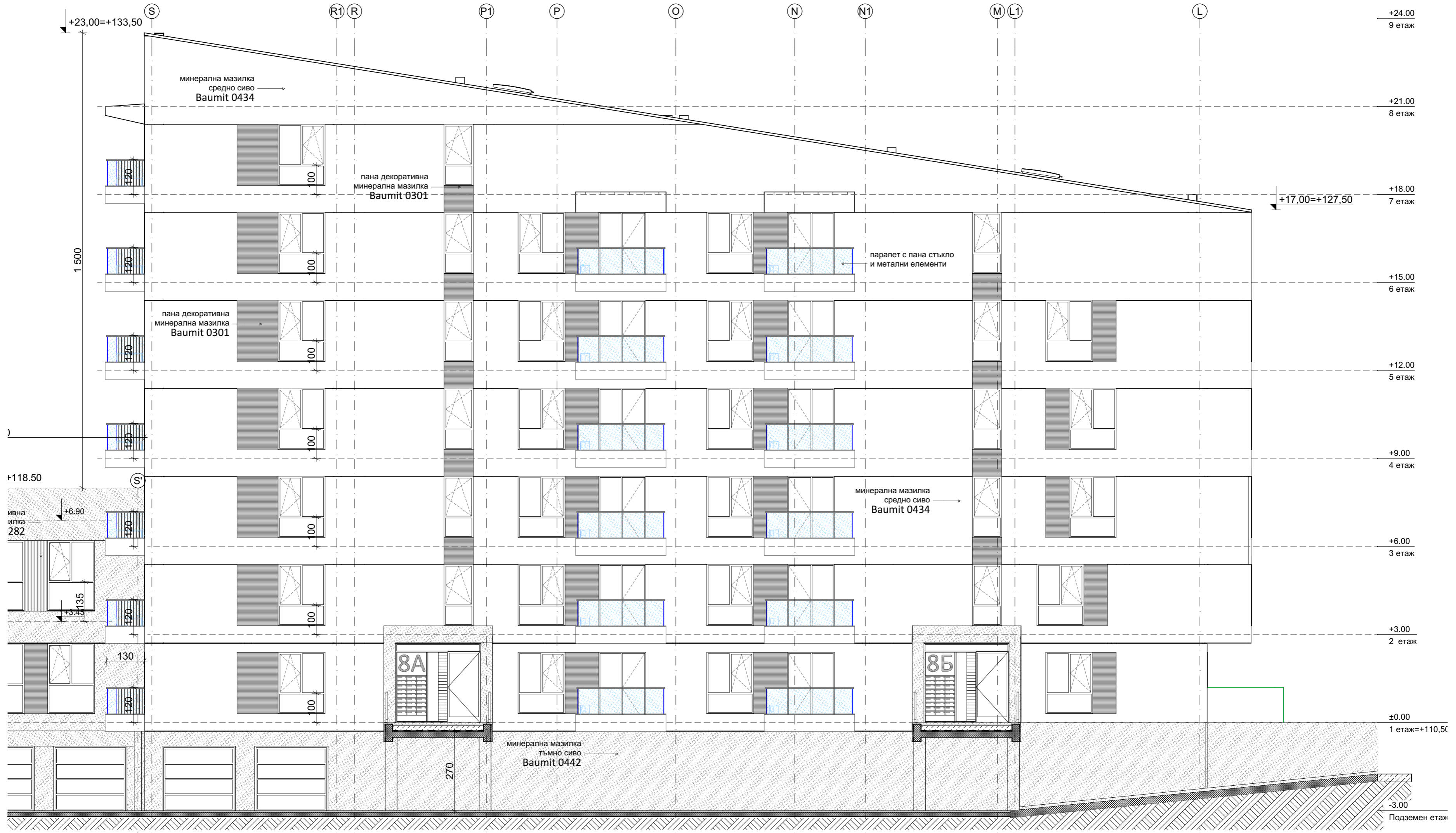
Фасада Север
