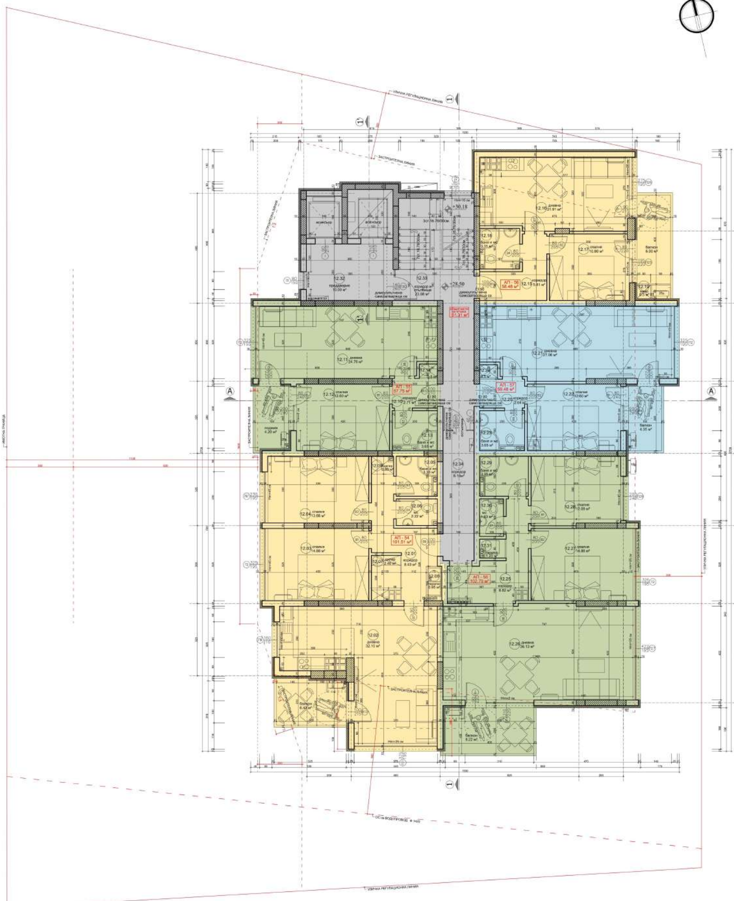
ЭТАЖ 12 РАЗПРЕДЕЛЕНИЕ НА КОТА +28.50 ЗП 441.32 м²
