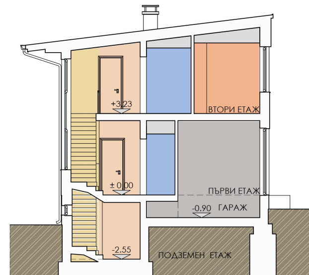
ВЕРТИКАЛЕН РАЗРЕЗ 1-1
