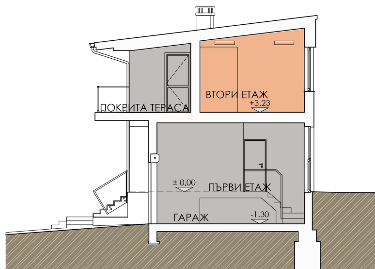
ВЕРТИКАЛЕН РАЗРЕЗ 1-1
