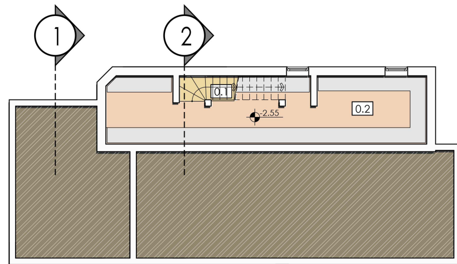
РАЗПРЕДЕЛЕНИЕ ПОДЗЕМЕН ЕТАЖ КОТА -2,55
