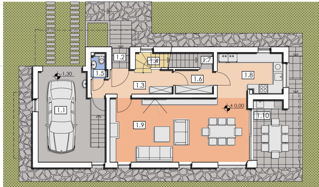
РАЗПРЕДЕЛЕНИЕ ПЪРВИ ЕТАЖ КОТИ -1,30 И ±0,00
