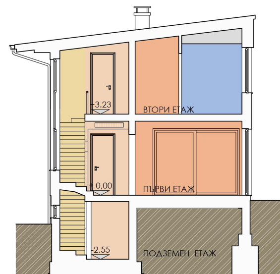
ВЕРТИКАЛЕН РАЗРЕЗ 2-2
