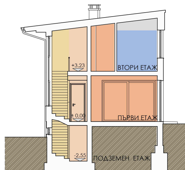
ВЕРТИКАЛЕН РАЗРЕЗ 2-2
