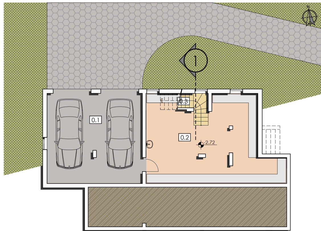
РАЗПРЕДЕЛЕНИЕ ПОЛУПОДЗЕМЕН ЕТАЖ КОТА -2,72
