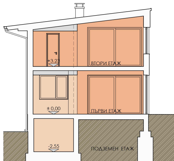
ВЕРТИКАЛЕН РАЗРЕЗ 2-2
