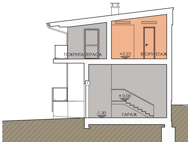
ВЕРТИКАЛЕН РАЗРЕЗ 1-1
