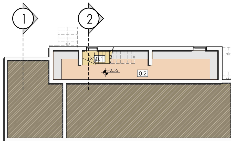
РАЗПРЕДЕЛЕНИЕ ПОДЗЕМЕН ЕТАЖ КОТА -2,55
