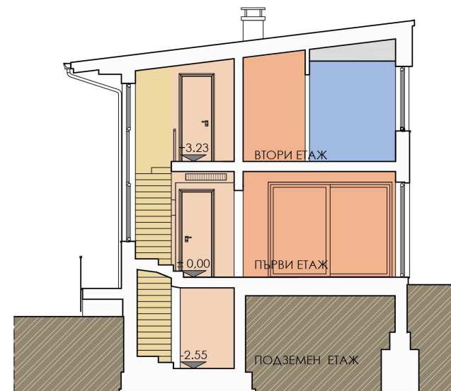
ВЕРТИКАЛЕН РАЗРЕЗ 2-2
