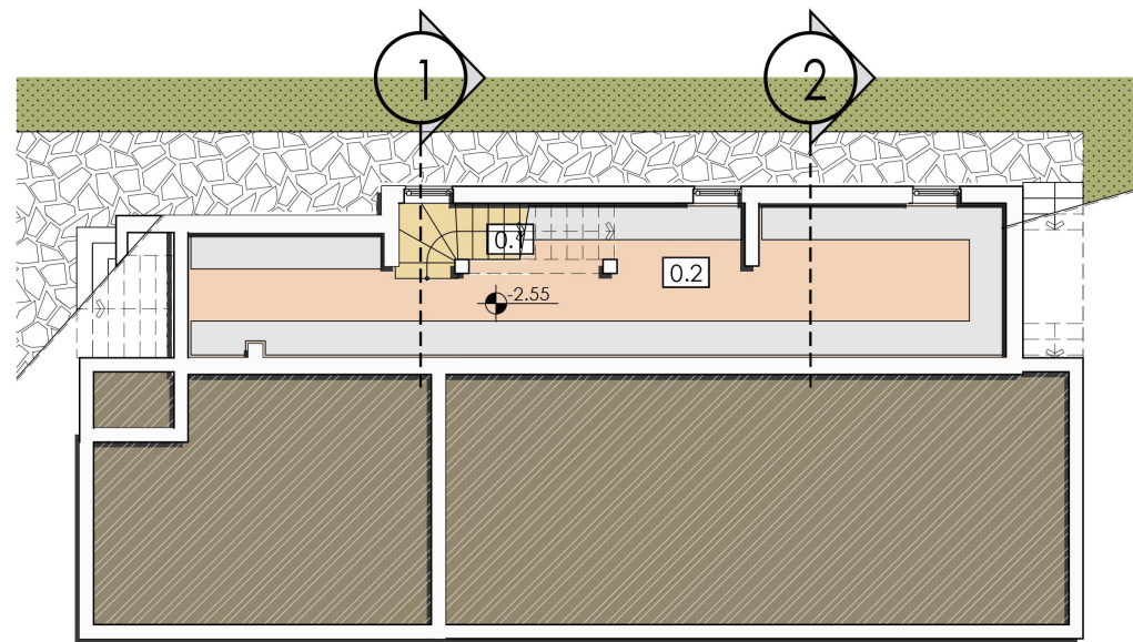
РАЗПРЕДЕЛЕНИЕ ПОДЗЕМЕН ЕТАЖ КОТА -2,55
