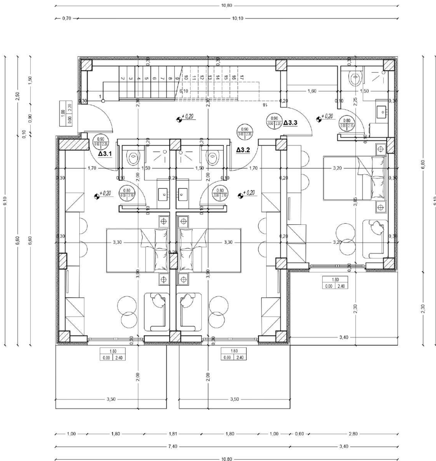
ΚΑΤΩΦΗ ΙΣΟΓΕΙΟΥ Κ3
