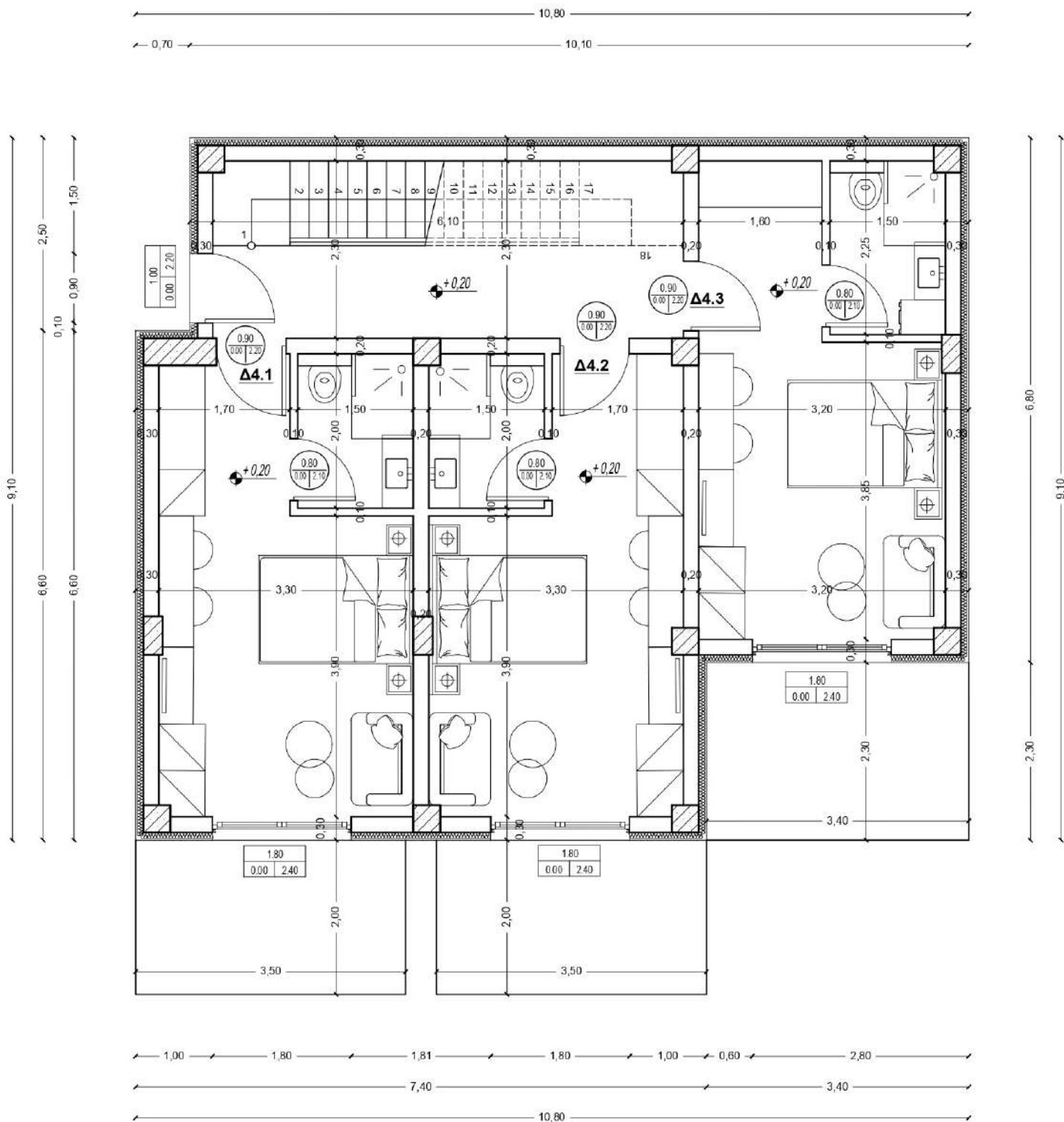
ΚΑΤΟΨΗ ΙΣΟΓΕΙΟΥ Κ4
