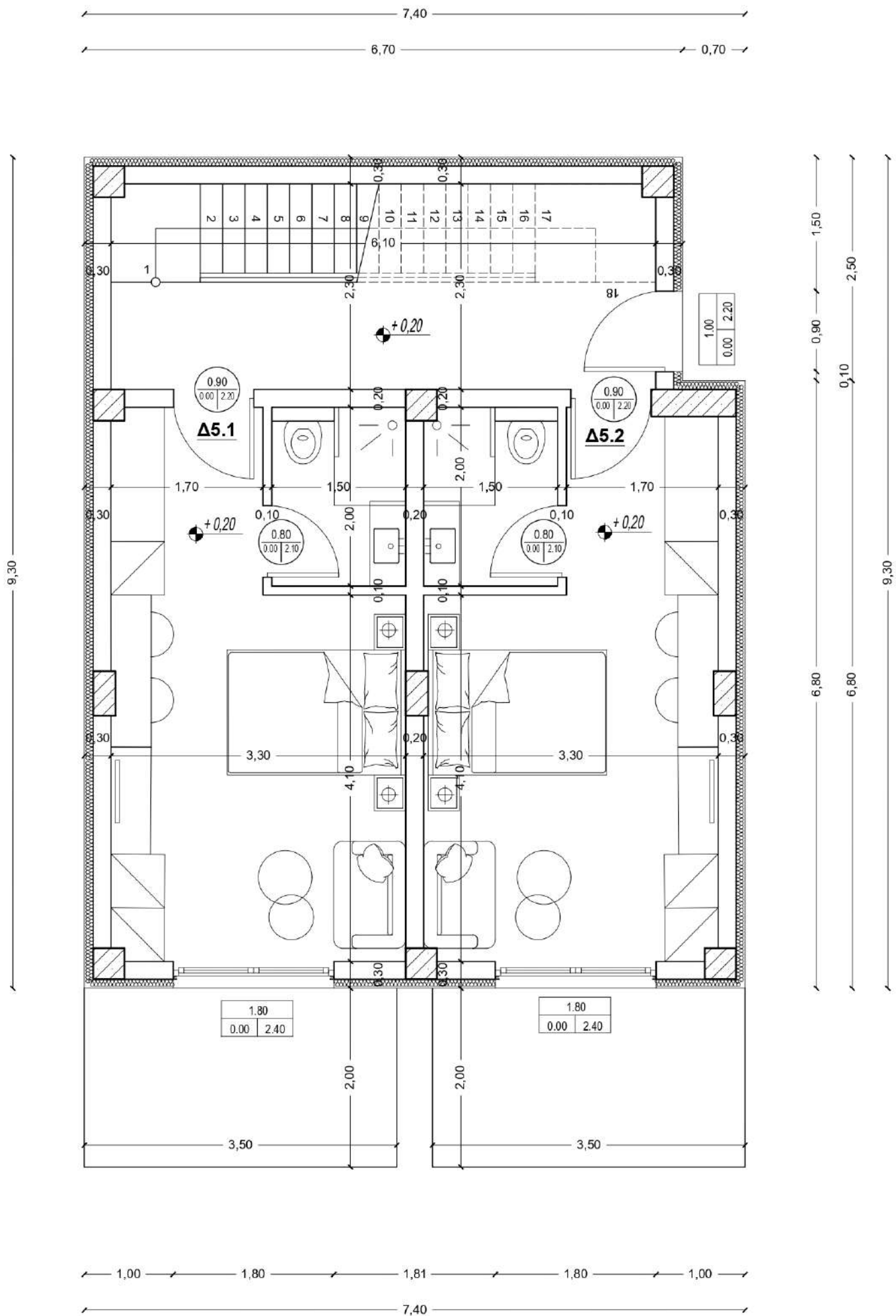
ΚΑΤΟΨΗ ΙΣΟΓΕΙΟΥ Κ5
