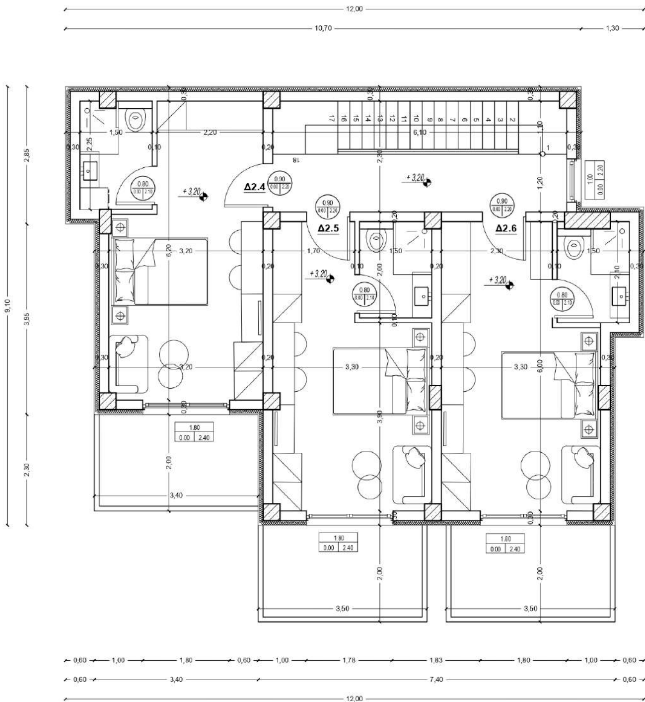
ΚΑΤΟΨΗ ΟΡΟΦΟΥ Κ2
