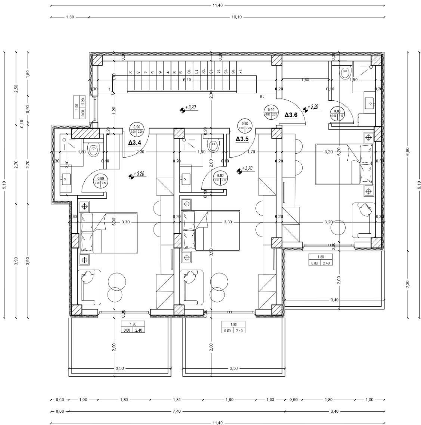
ΚΑΤΟYΗ ΟΡΟΦΟΥ Κ3
