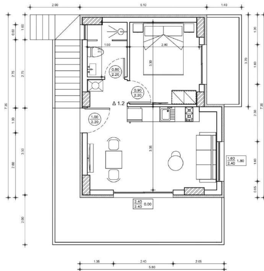
ΚΑΤΟΨΗ Α ΟΡΟΦΟΥ ΚΤΙΡΙΟΥ 1
