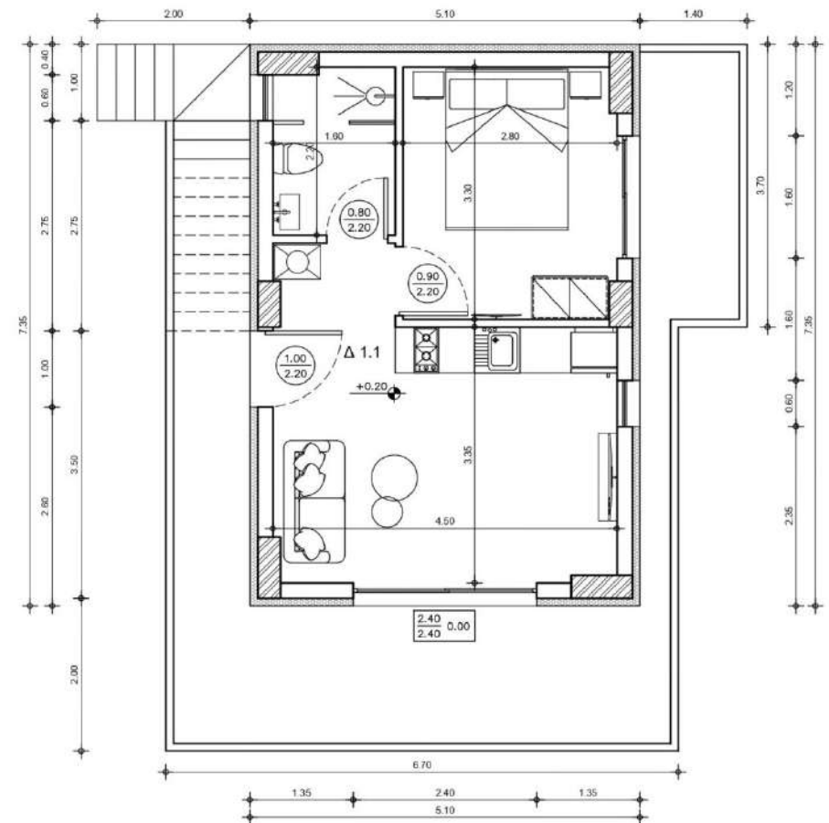
ΚΑΤΟΨΗ ΙΣΟΓΕΙΟΥ ΚΤΙΡΙΟΥ 1
