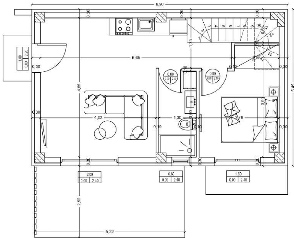
ΚΑΤΟΨΗ ΙΣΟΓΕΙΟΥ
