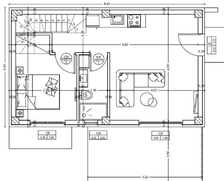
ΚΑΤΩΦΗ ΙΣΟΓΕΙΟΥ
