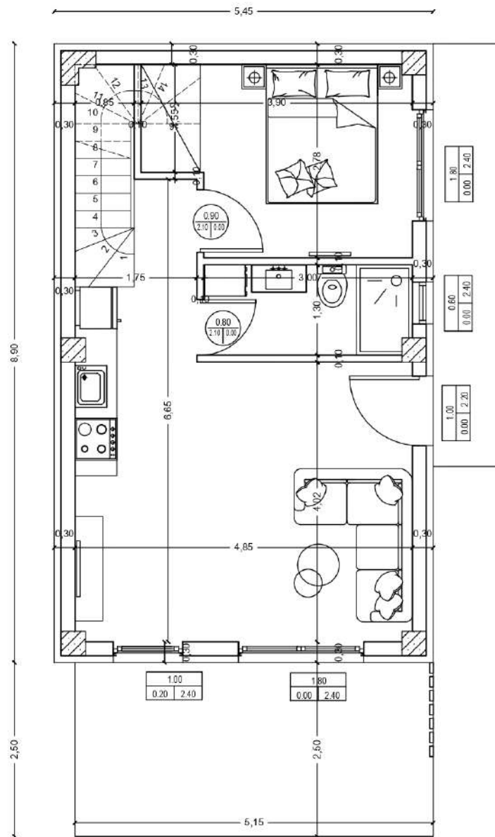
ΚΑΤΟΨΗ ΙΣΟΓΕΙΟΥ
