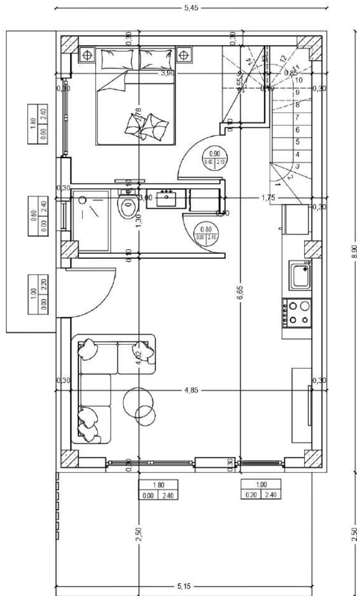
ΚΑΤΟΨΗ ΙΣΟΓΕΙΟΥ
