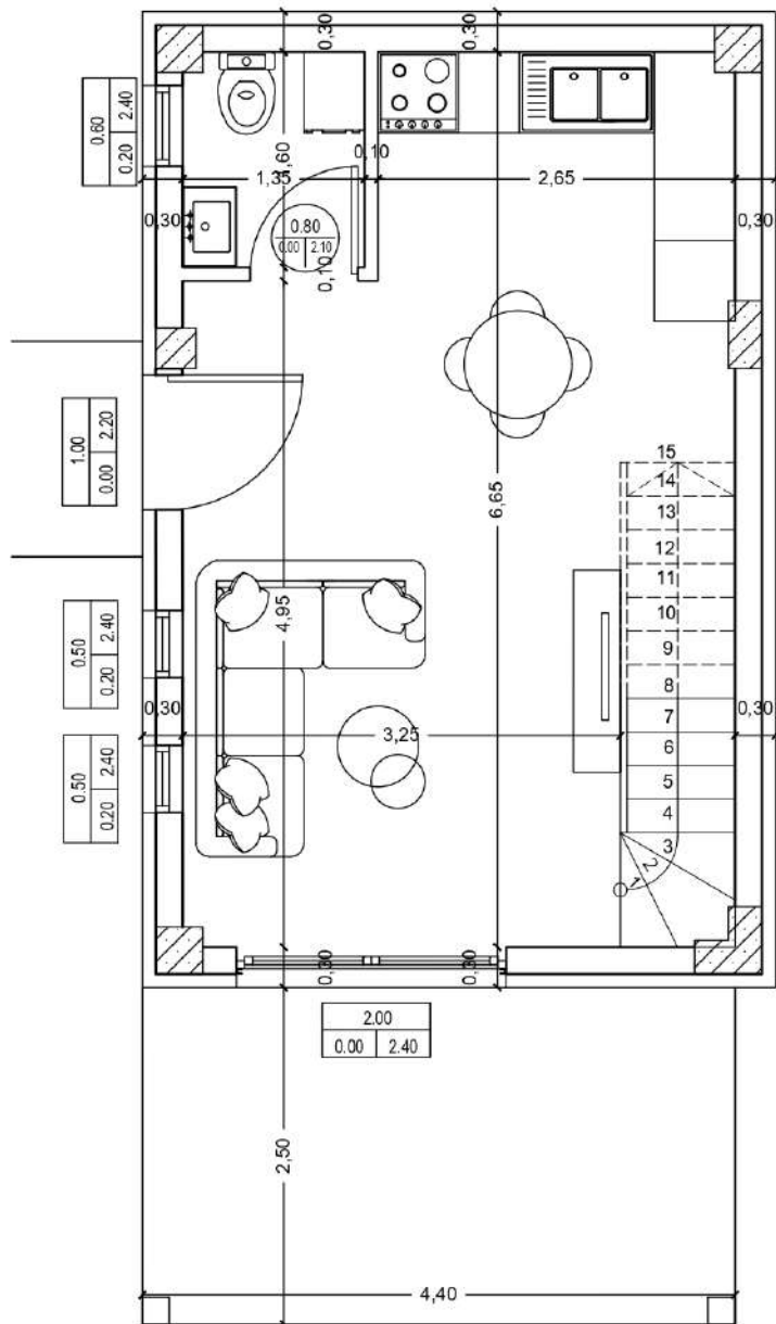
ΚΑΤΟΨΗ ΙΣΟΓΕΙΟΥ
