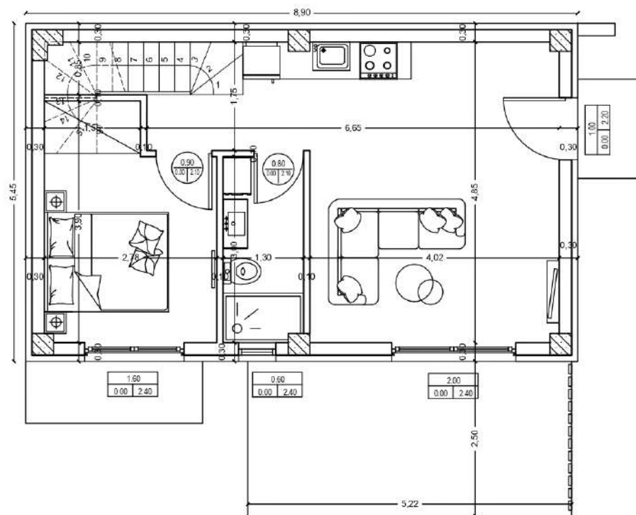
ΚΑΤΩΦΗ ΙΣΟΓΕΙΟΥ
