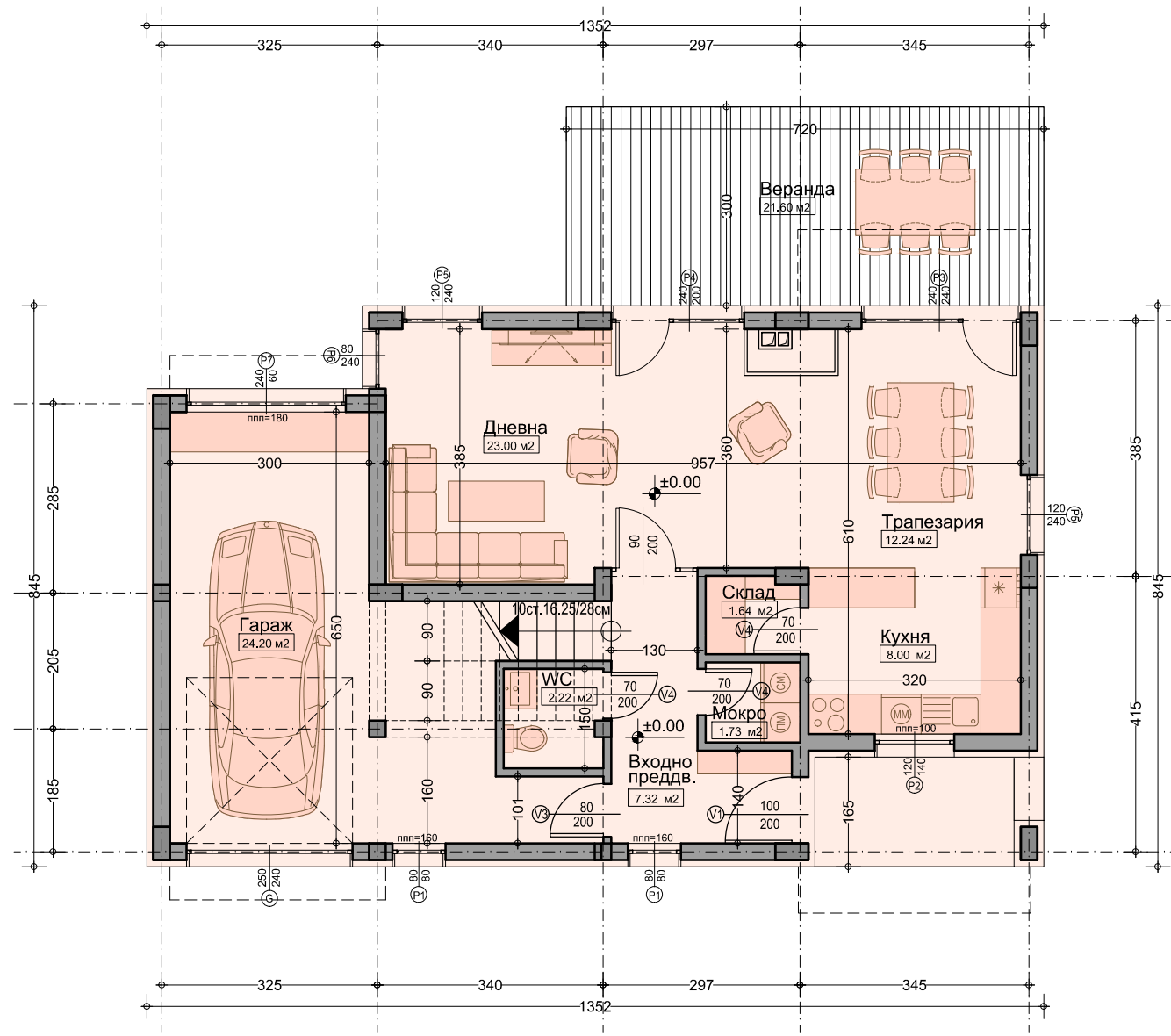
РАЗПРЕДЕЛЕНИЕ ПЪРВИ ЕТАЖ М 1:100 ЗАСТРОЕНА ПЛОЩ: 110.18м²
