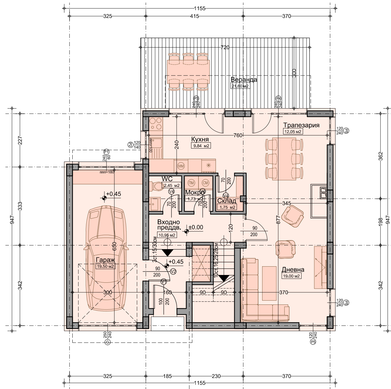
РАЗПРЕДЕЛЕНИЕ ПЪРВИ ЕТАЖ М 1:100 ЗАСТРОЕНА ПЛОЩ: 101.16м²
