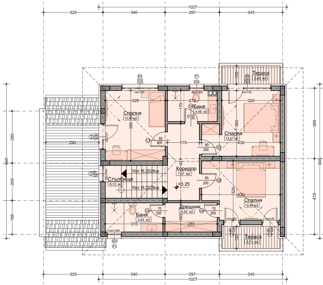
РАЗПРЕДЕЛЕНИЕ ВТОРИ ЕТАЖ М 1:100 ЗАСТРОЕНА ПЛОЩ: 93.27м²
