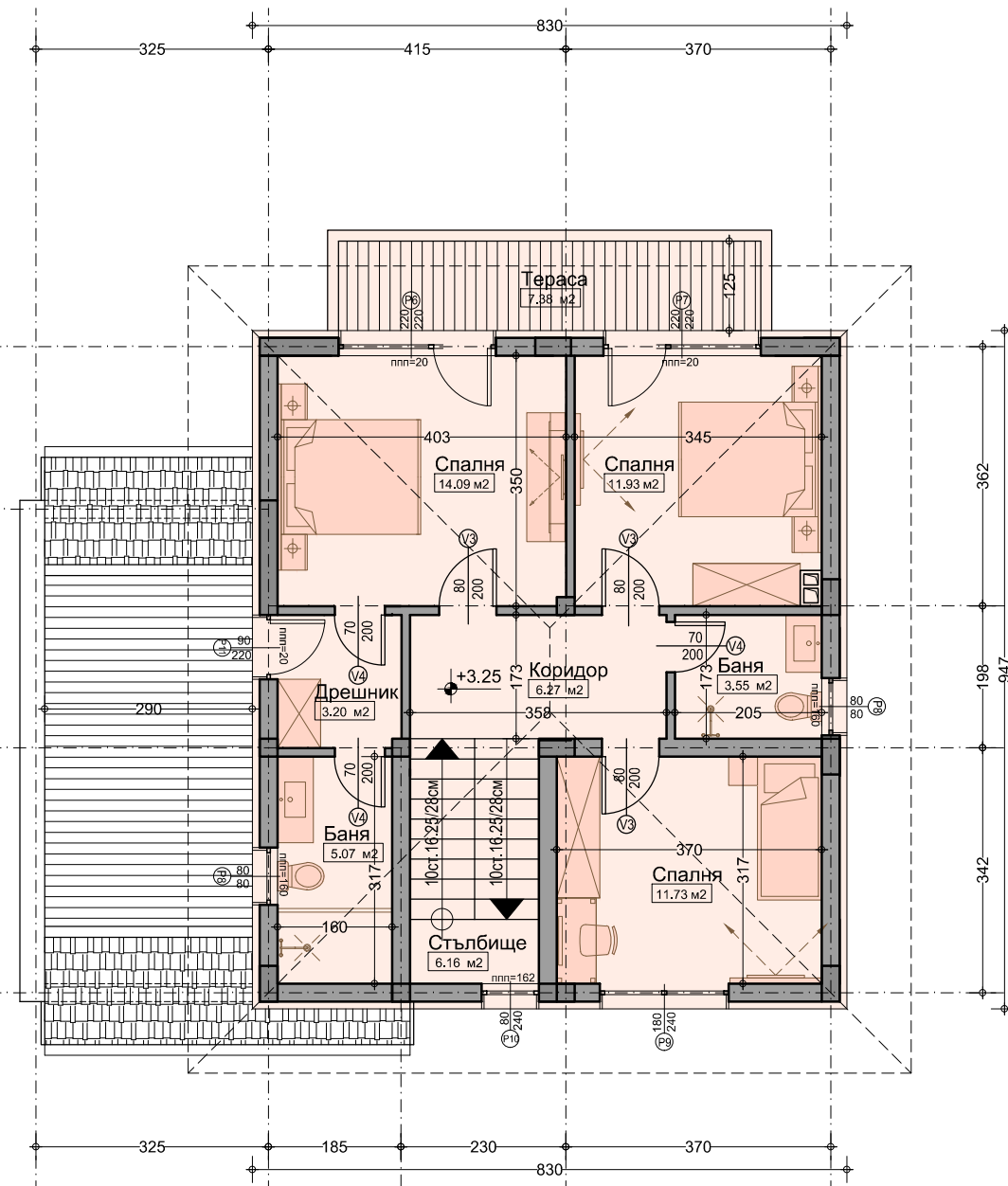
РАЗПРЕДЕЛЕНИЕ ВТОРИ ЕТАЖ М 1:100 ЗАСТРОЕНА ПЛОЩ: 87.28м²
