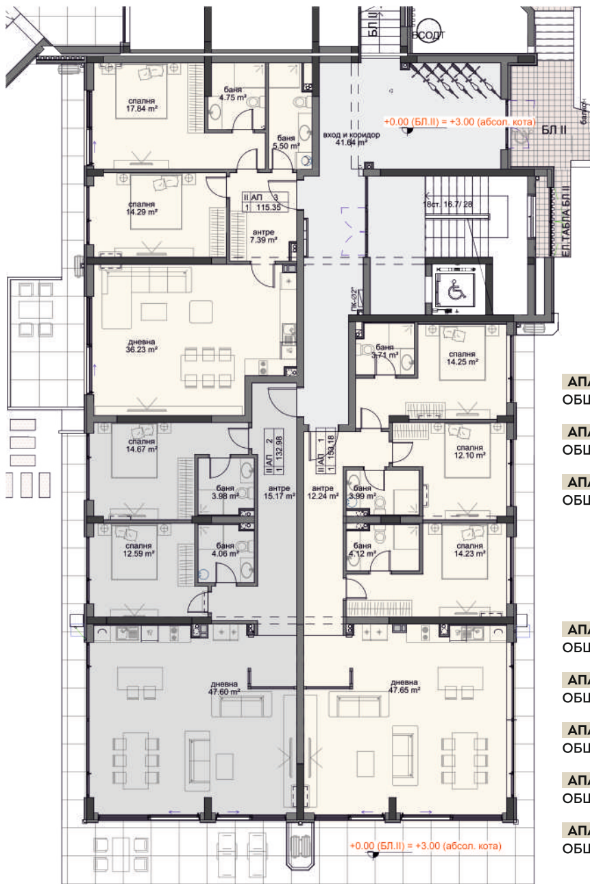
Разпределение етаж 1
