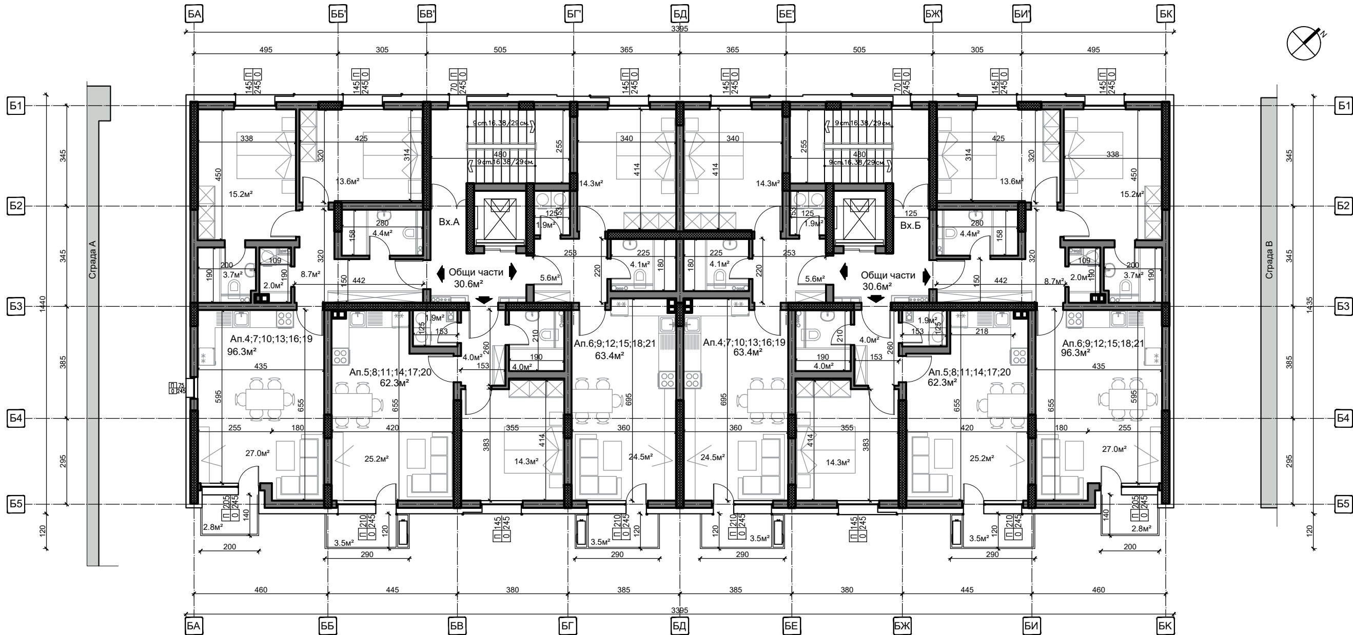
Сграда Б - Разпределение на типов етаж (2-7 етаж)
